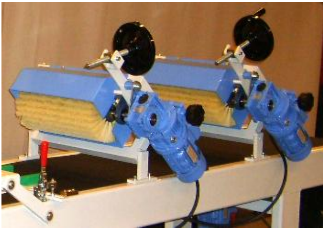
Optie: extra borstel aan uitvoerzijde.
