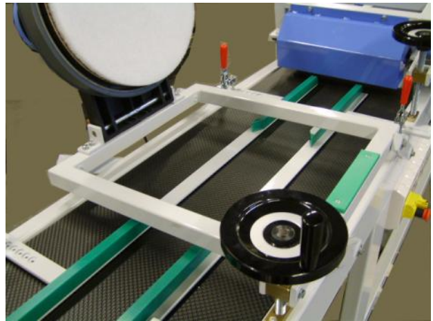
Zijgeleiding uit 1 deel voor kleine parketdelen.
